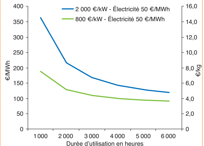
Fig. 5 – Coûts de production de l'hydrogène en fonction des investissements et de la durée d'utilisation de l'électrolyseur
