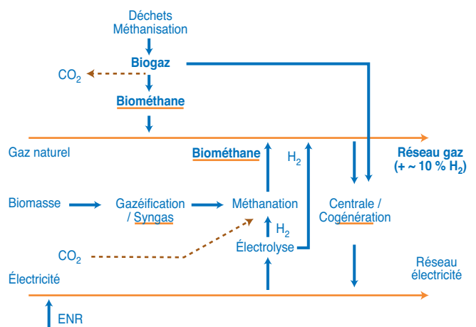
Fig. 2 – Intégration du biogaz et du biométhane dans un schéma global gaz/électricité/hydrogène
